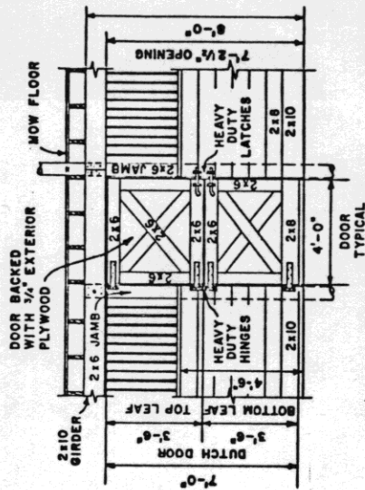
ELEVATION C-C SCALE: 1/4"=1'-0"
