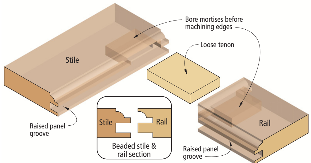
Door construction
